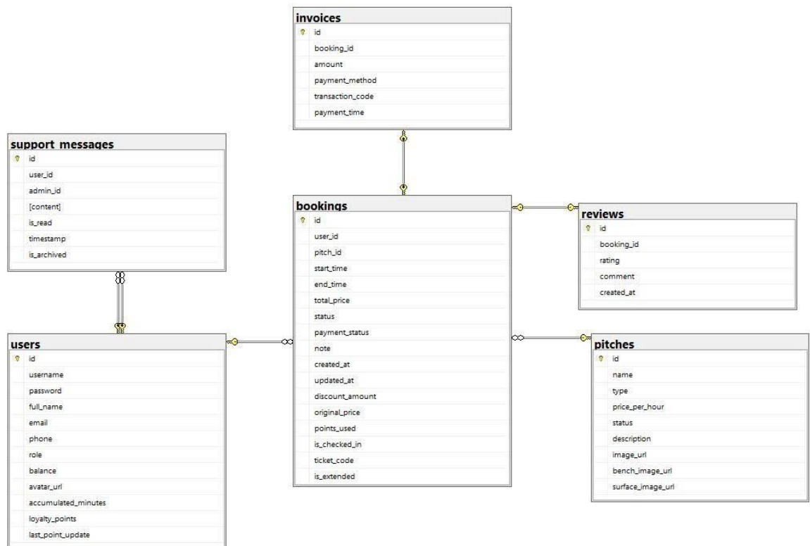
Hình 42: Class Diagram
